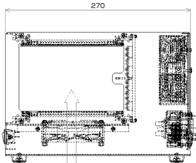
右側面図
