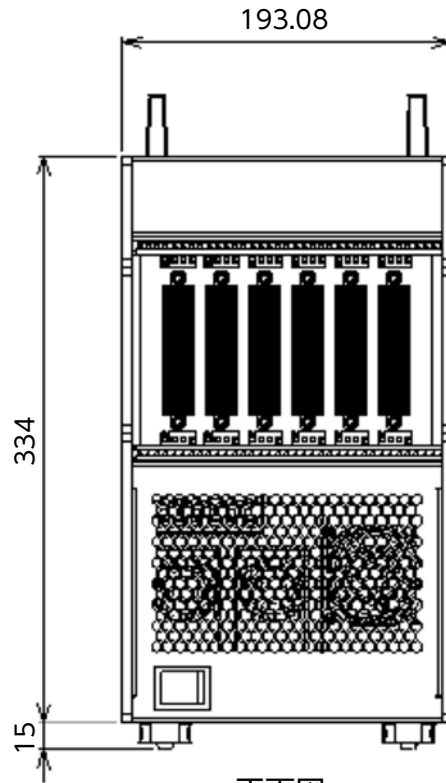
正面図
