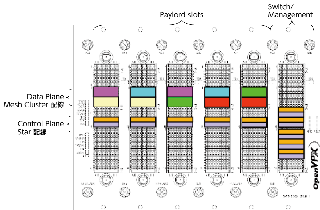
バックプレーン接続概要
