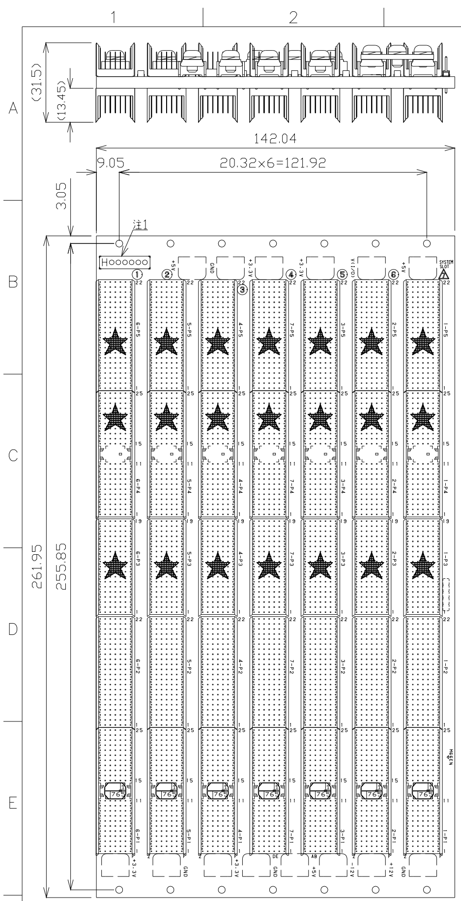
部品面視
