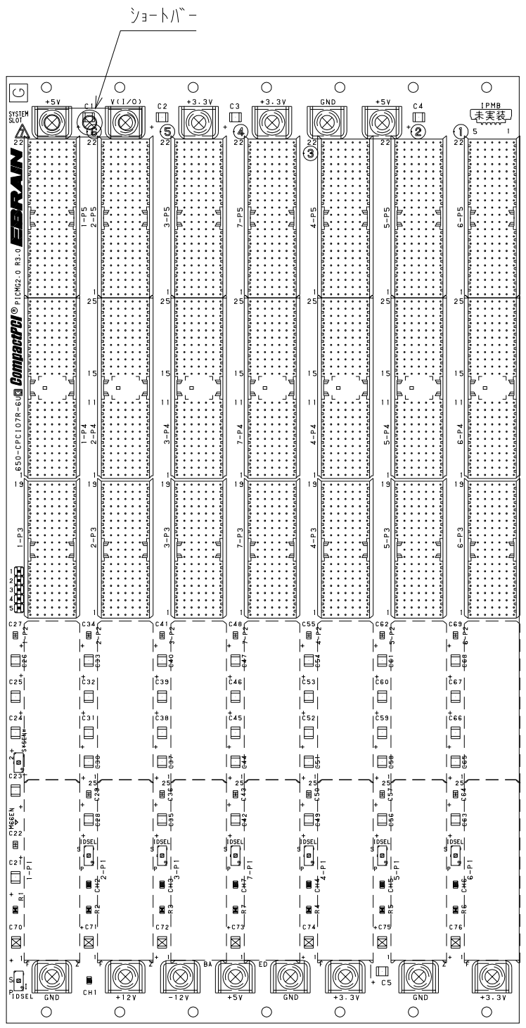
半田面視
