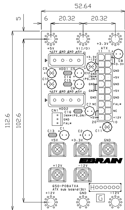
部品面視
