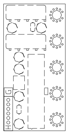
半田面視
