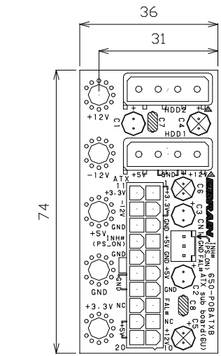
部品面視
