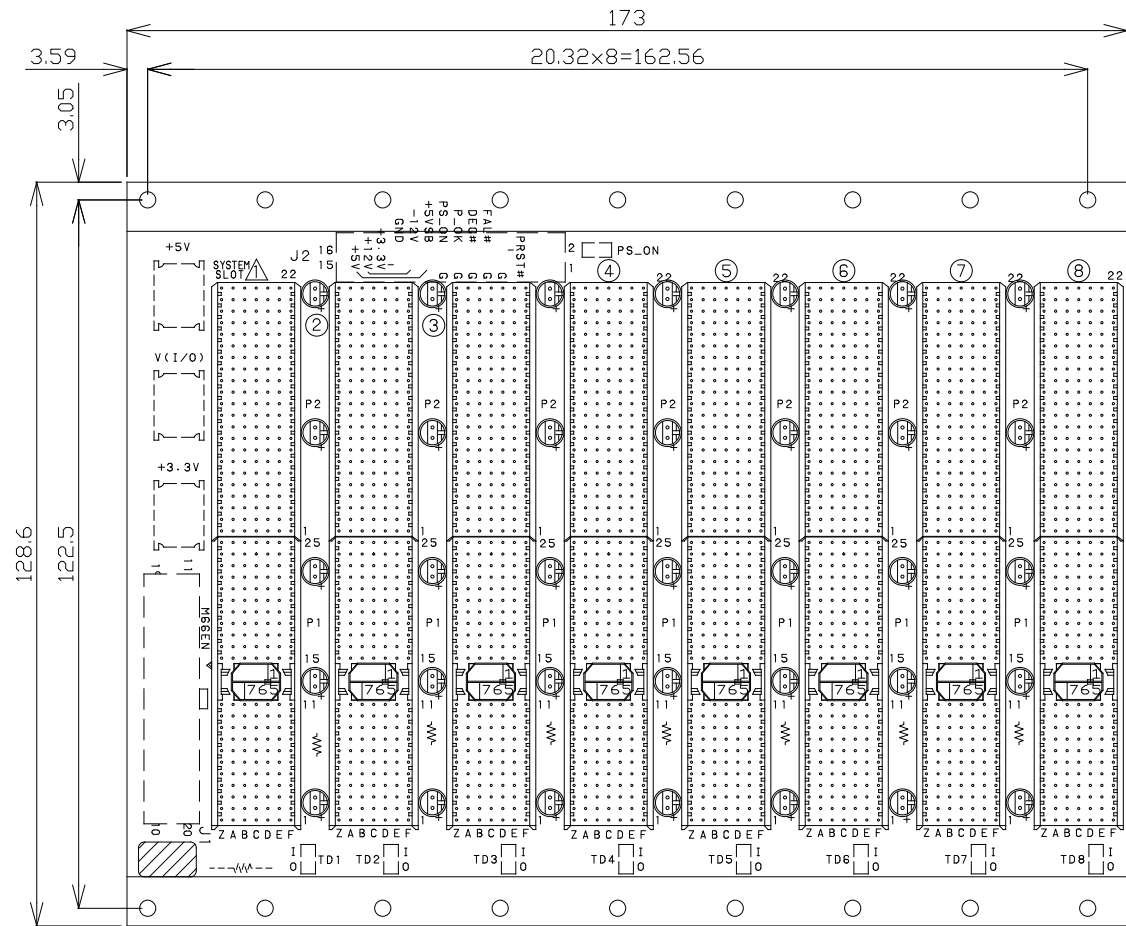
部品面視
