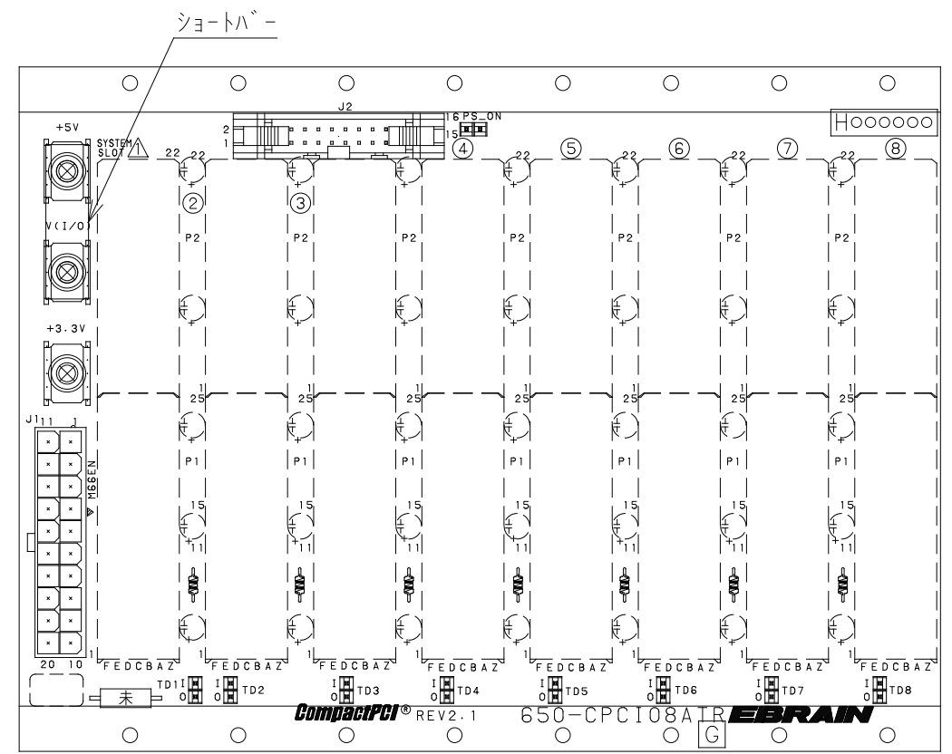
半田面視
