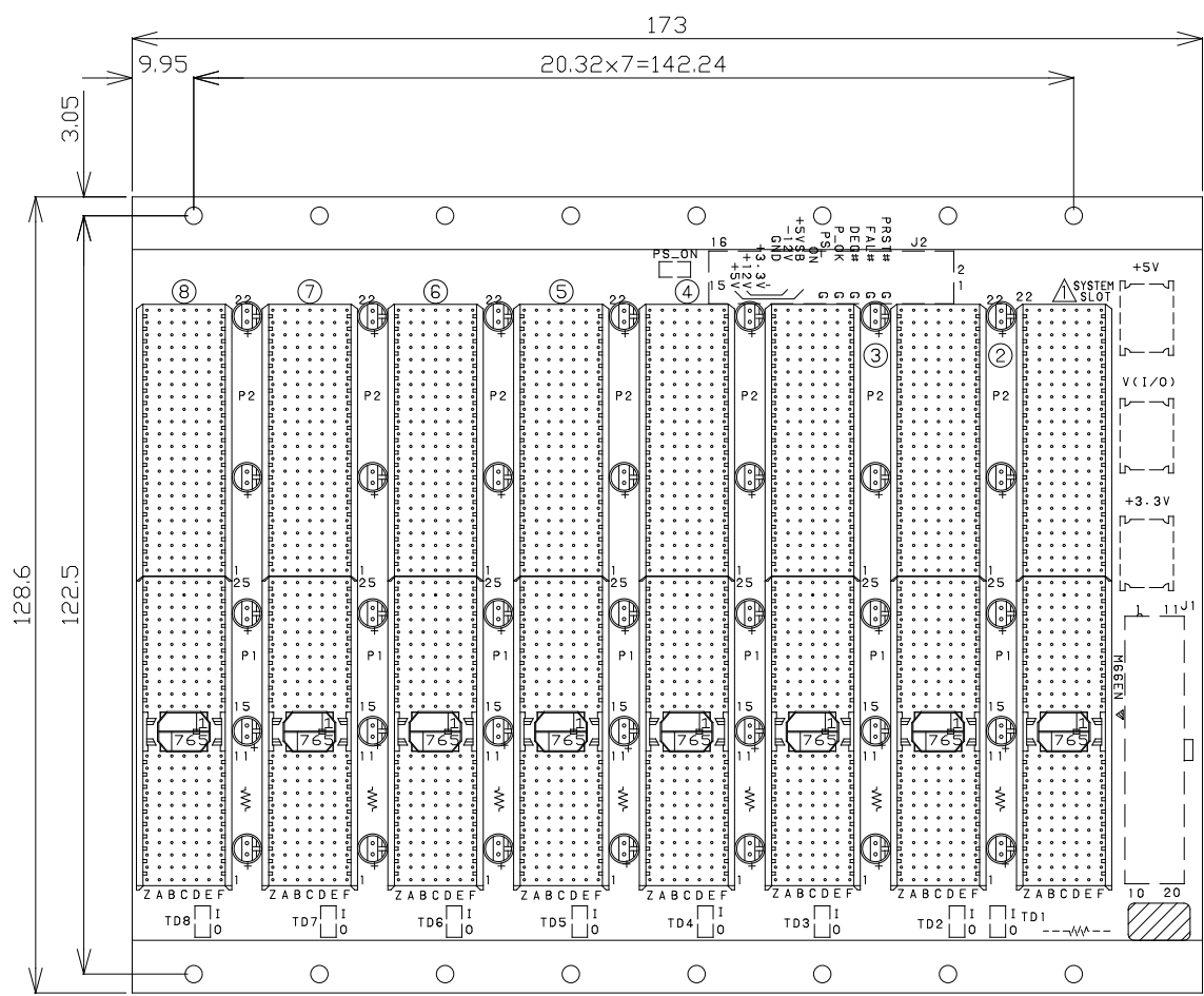
部品面視
