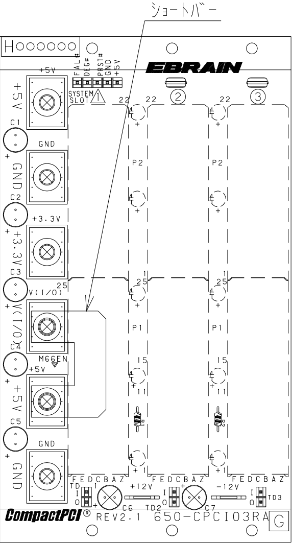
半田面視
