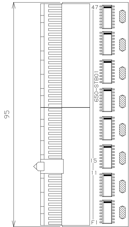
部品面視
