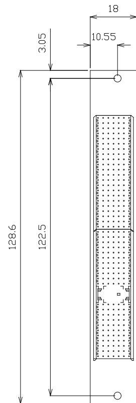
部品面視
