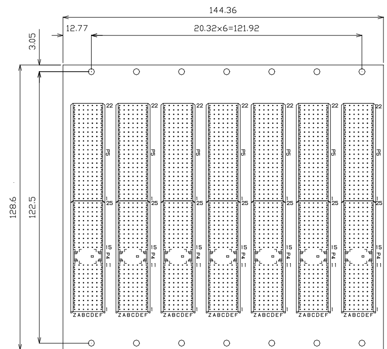
部品面視
