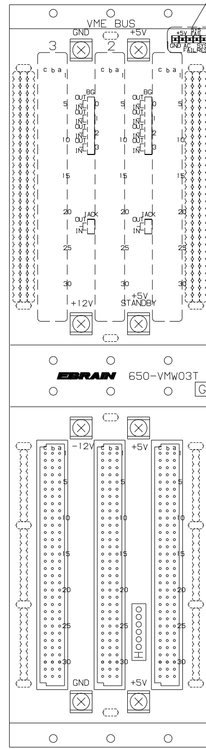
半田面視
