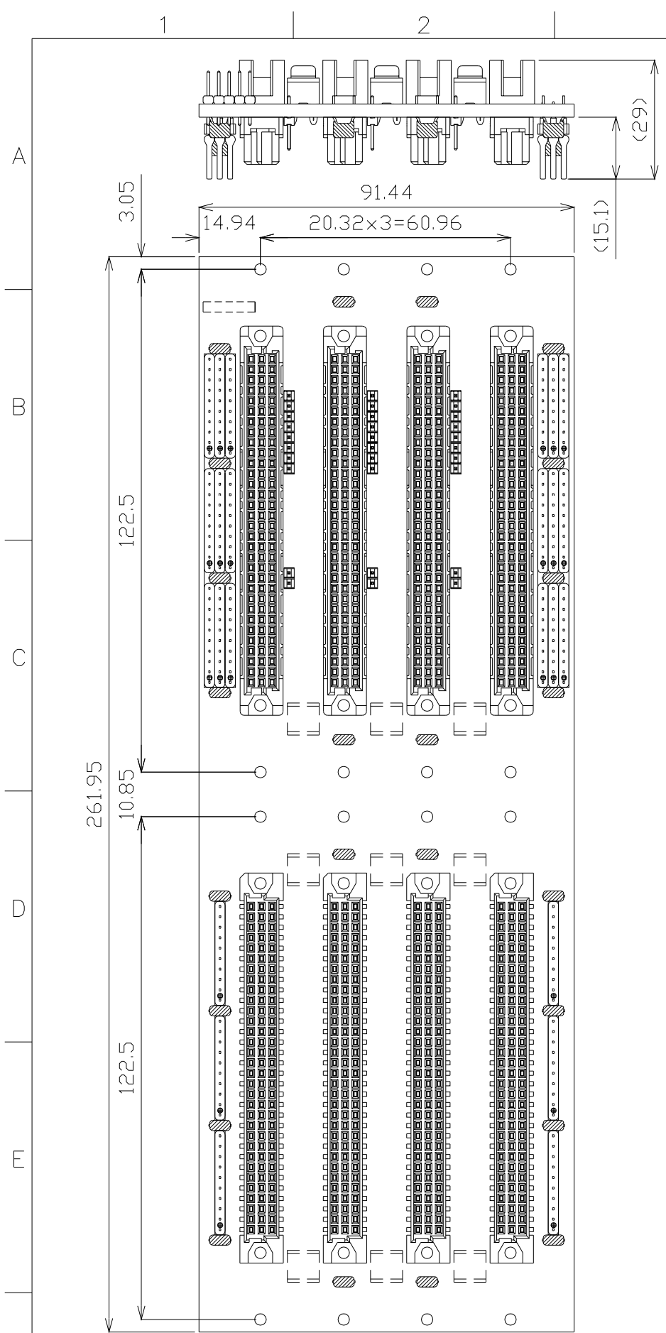
部品面視
