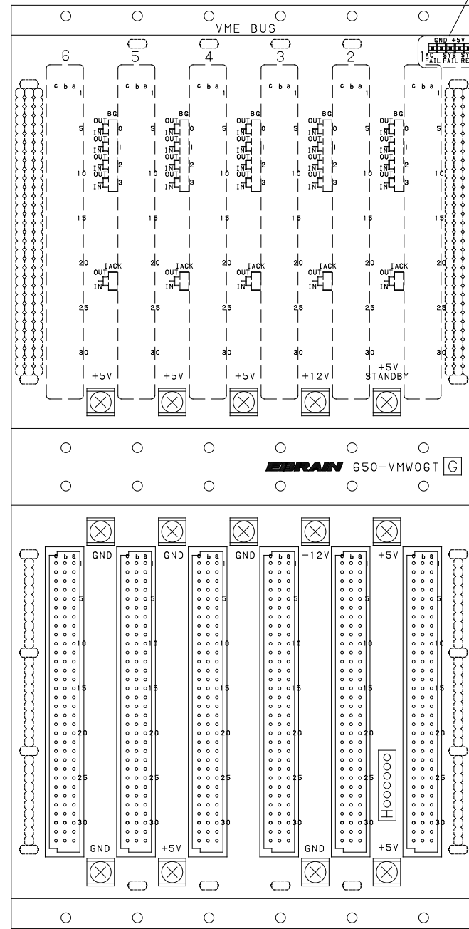
半田面視
