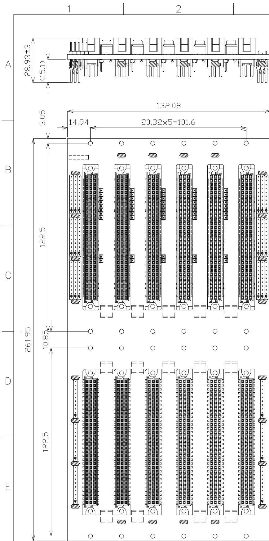
部品面視
