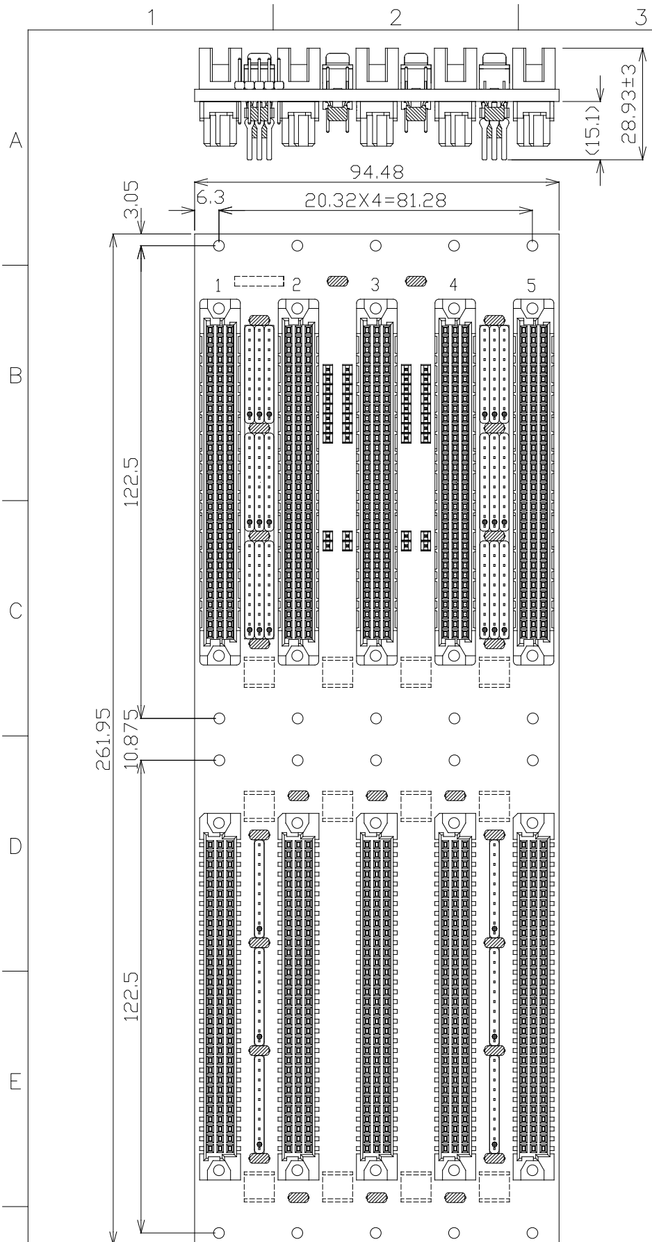
部品面視
