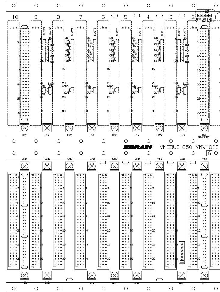
半田面視
