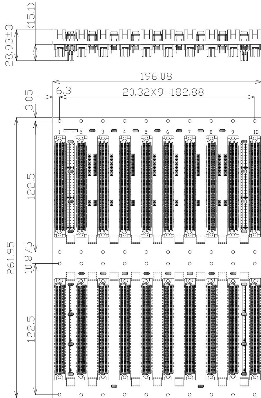
部品面視
