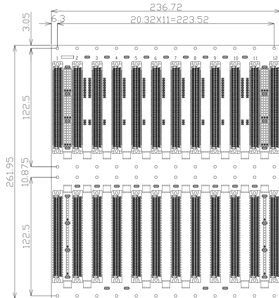
部品面視
