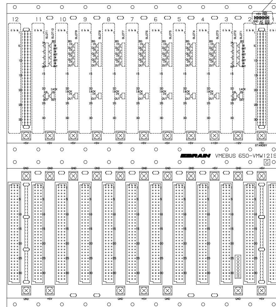
半田面視
