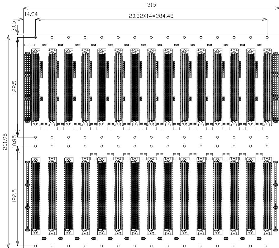
部品面視
