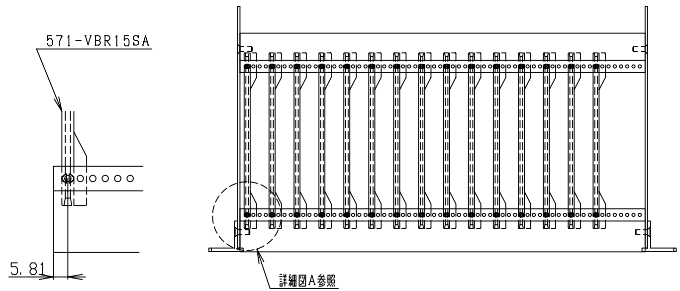
詳細図A
