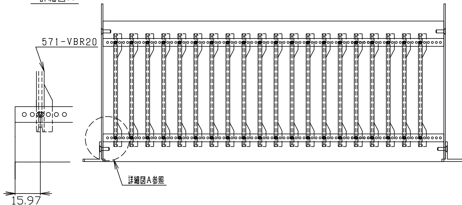
詳細図A
