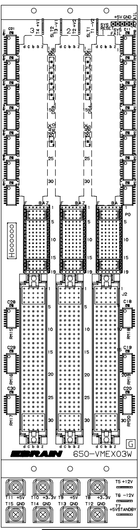
半田面視
