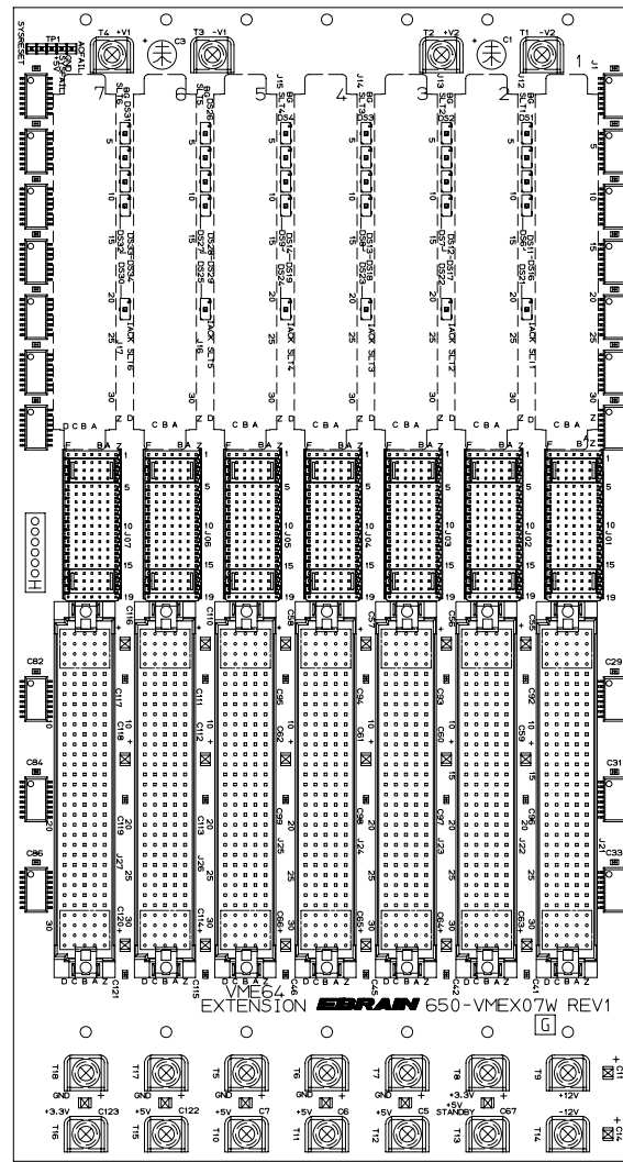
半田面視
