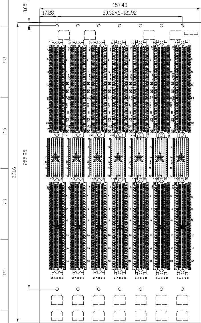
部品面視
