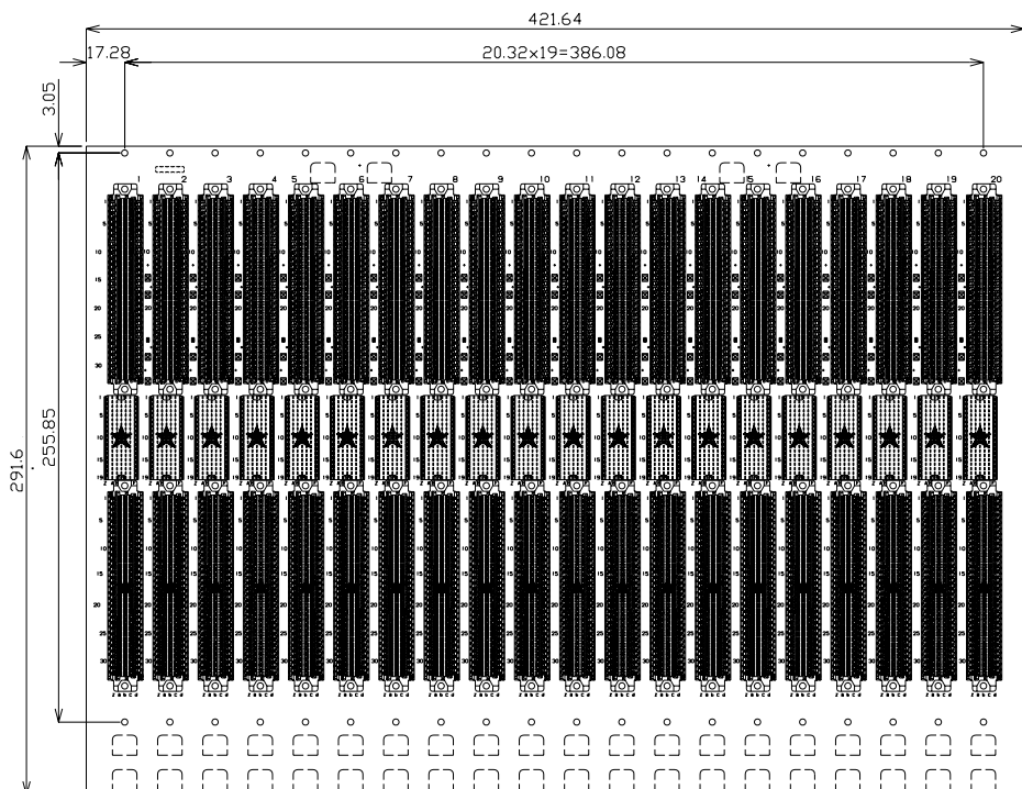
部品面視
