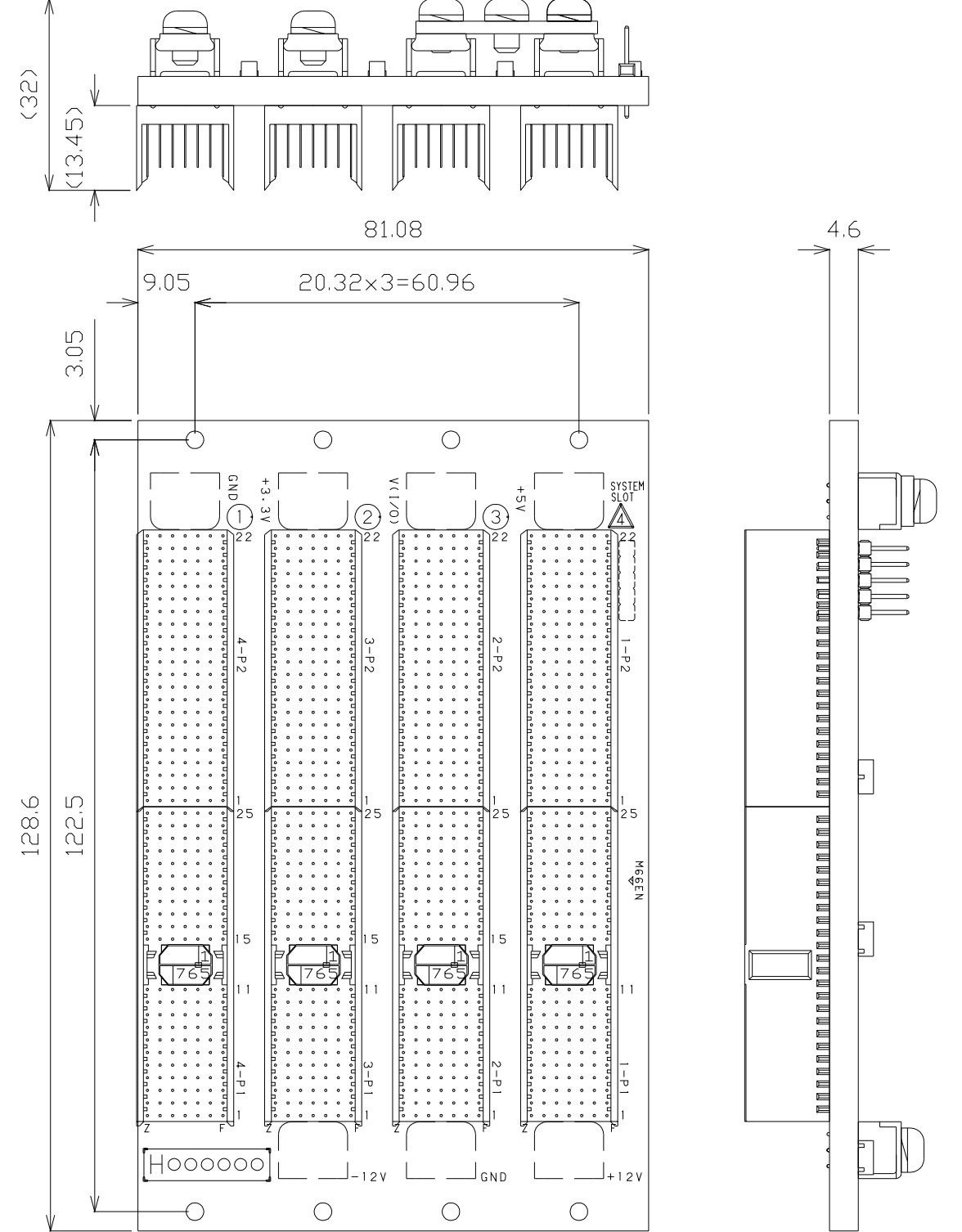
部品面視
