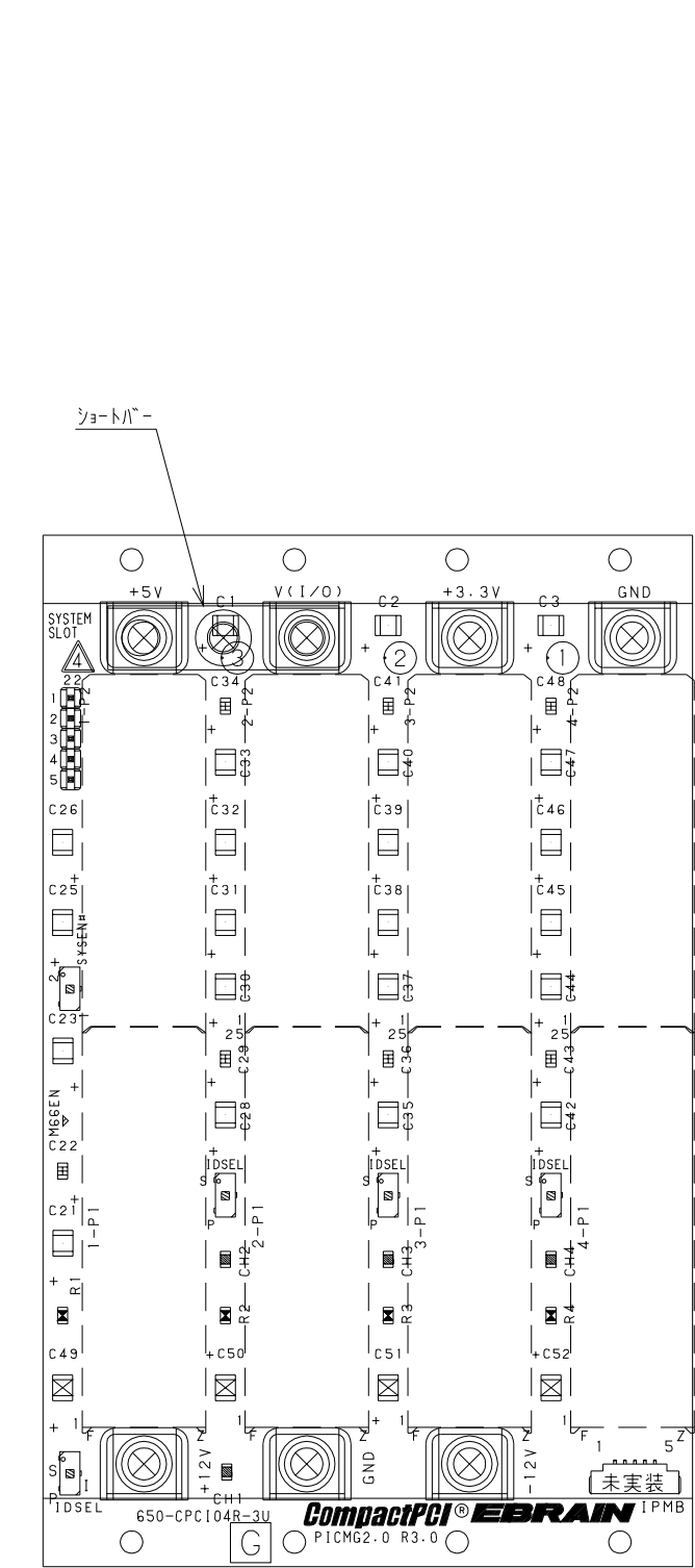
半田面視
