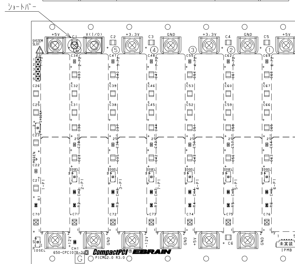
半田面視
