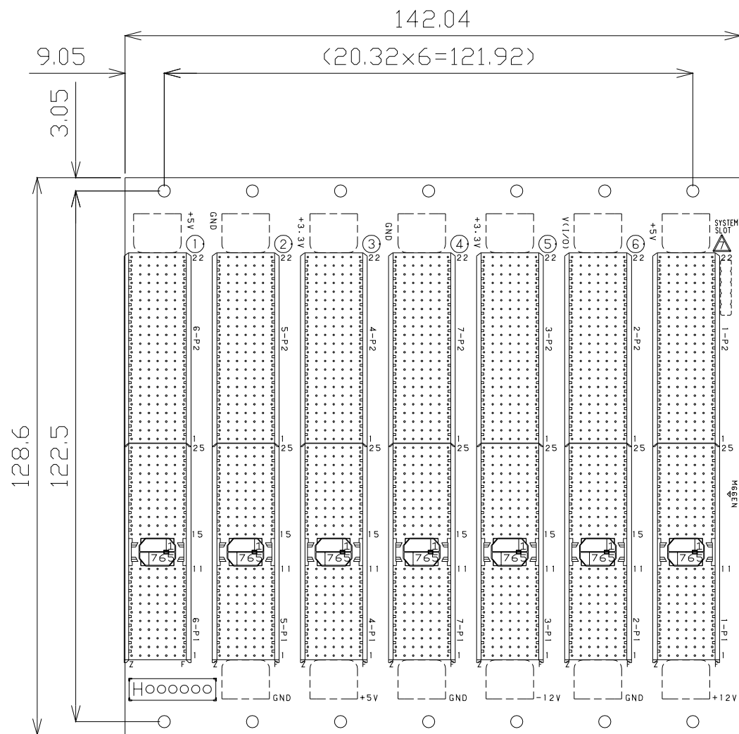
部品面視
