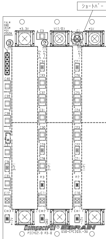
半田面視
