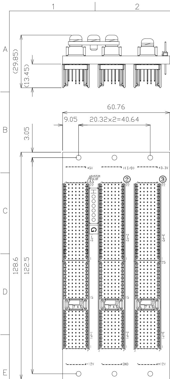
部品面視
