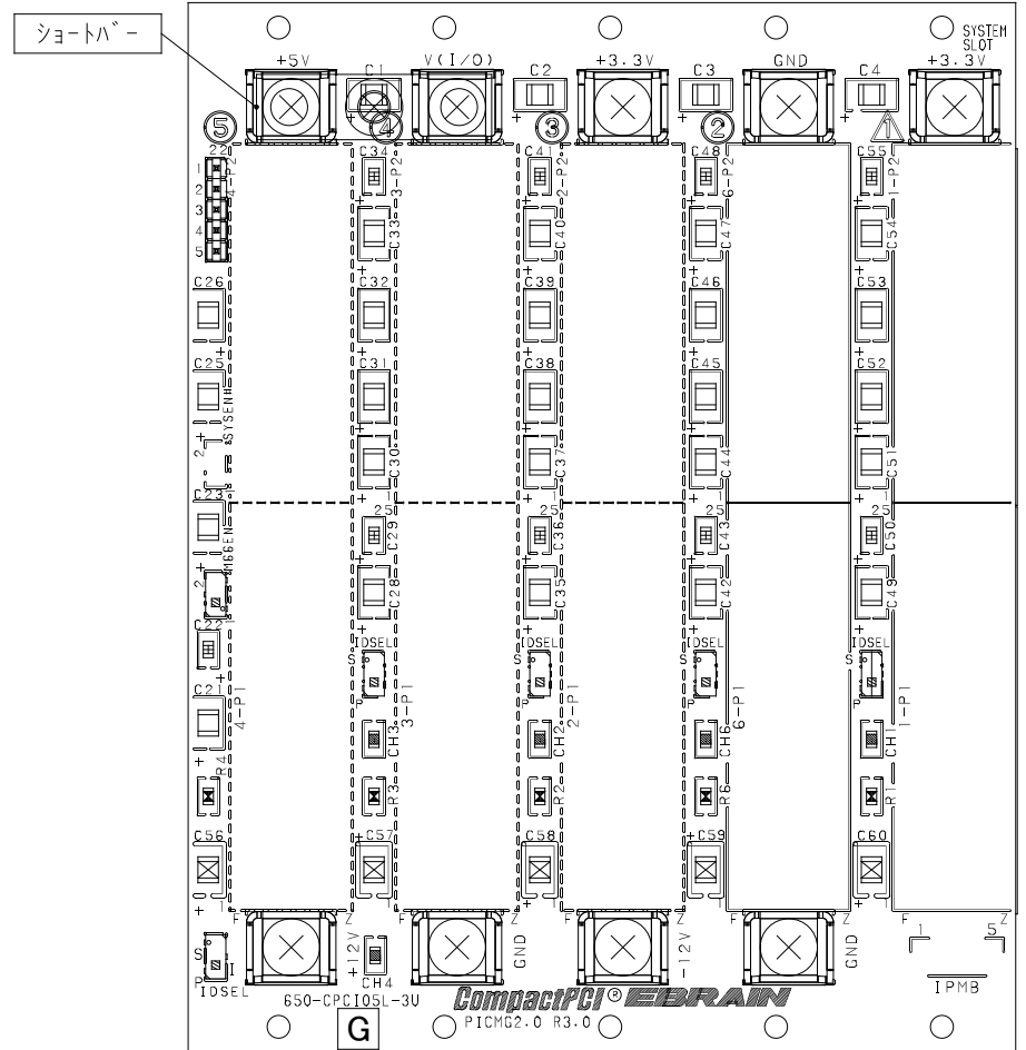
半田面視
