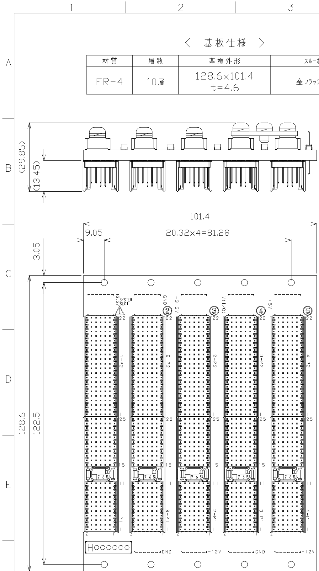
部品面視
