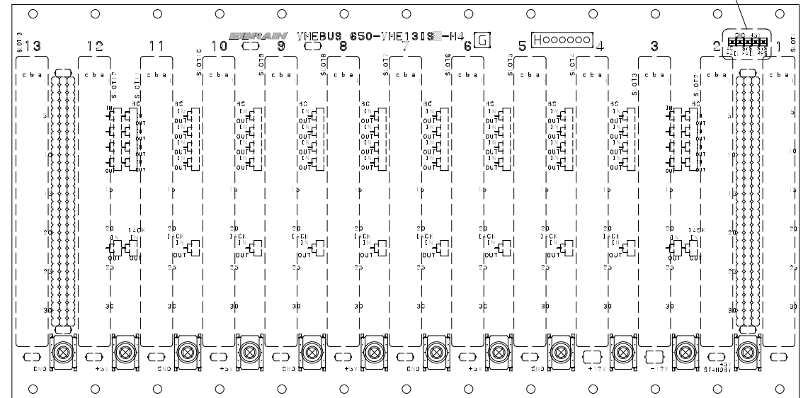
半田面視
