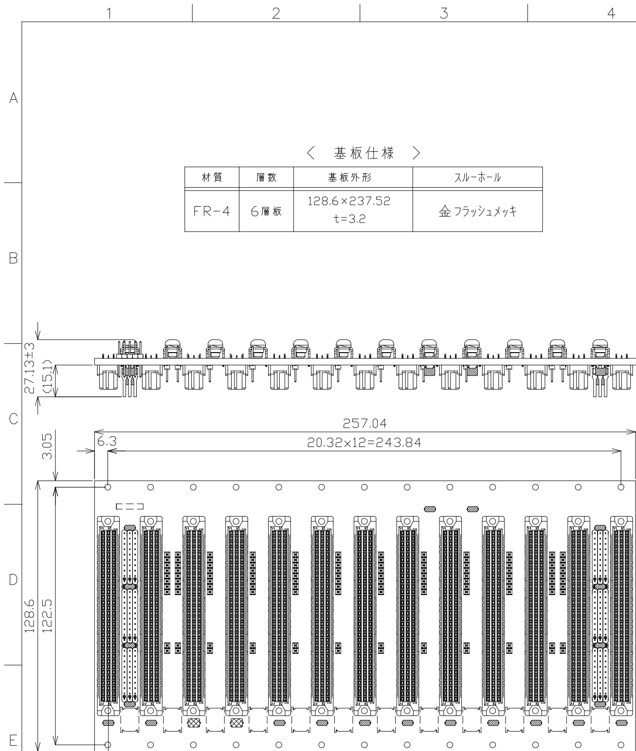
部品面視
