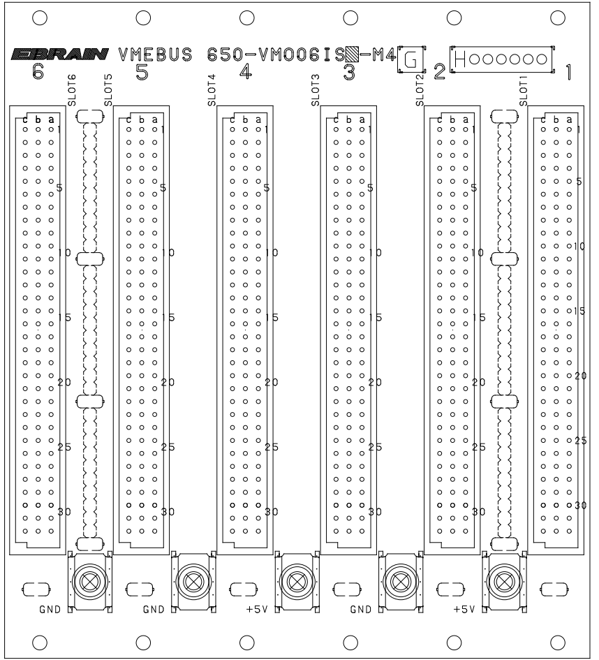
半田面視
