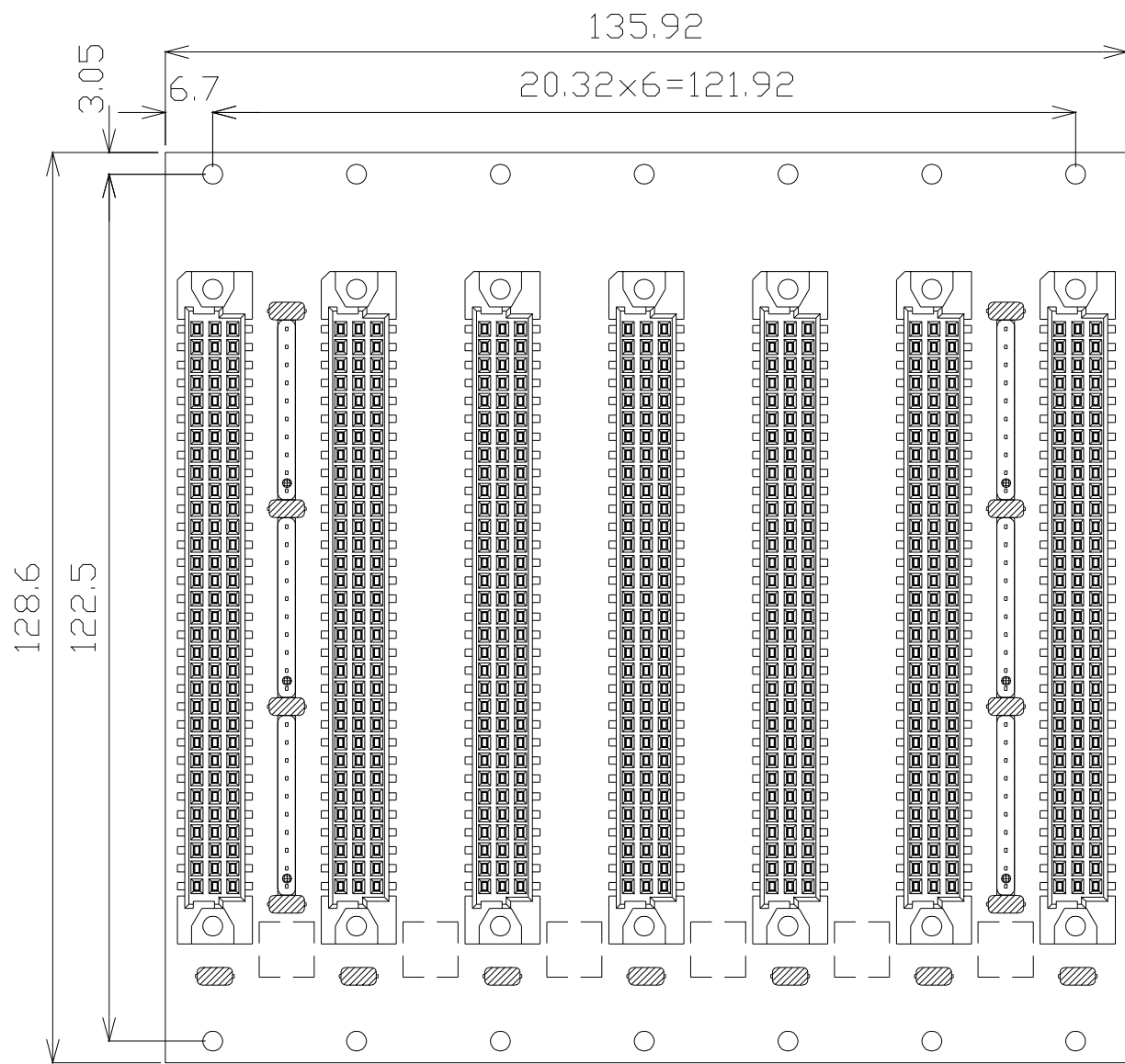
部品面視
