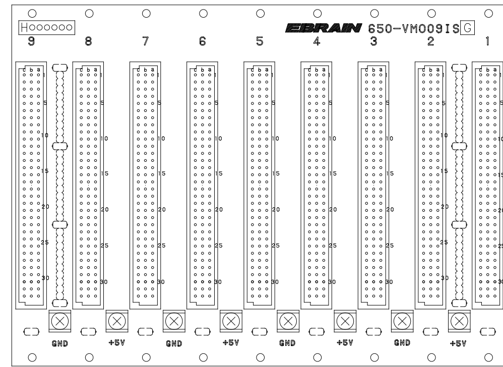
半田面視
