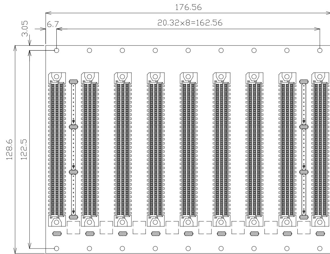
部品面視
