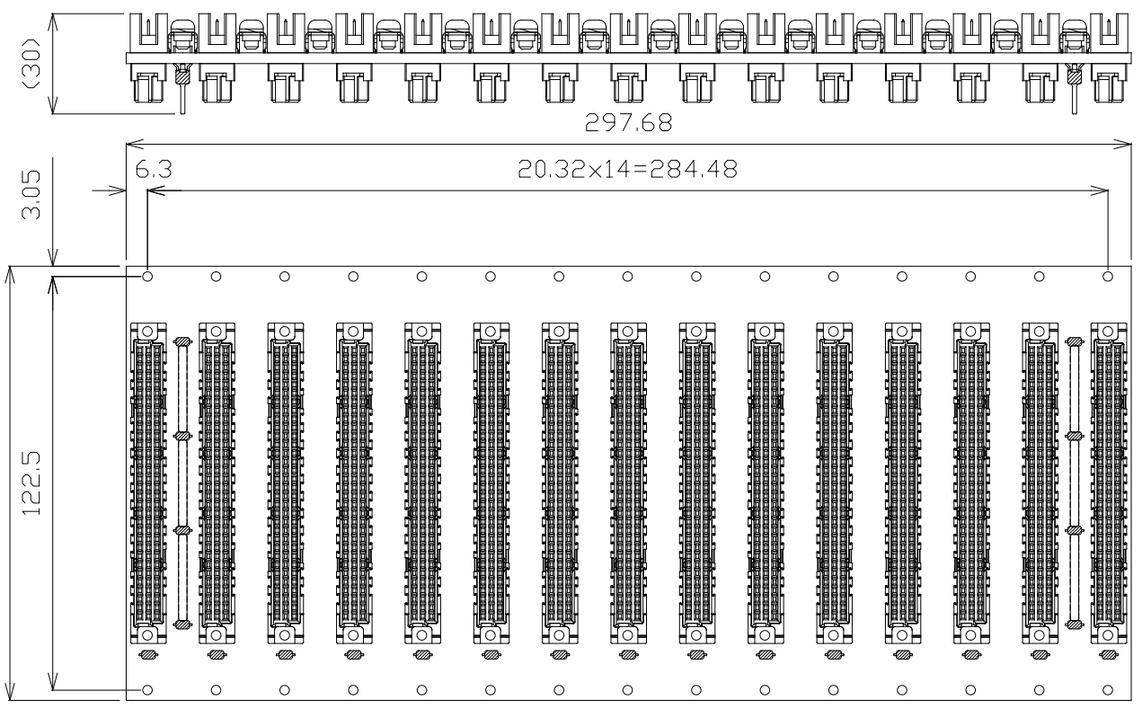
部品面視
