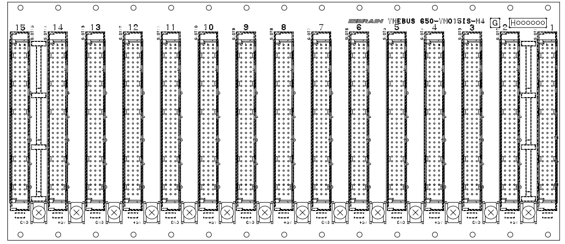
半田面視
