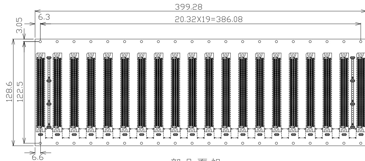
部品面視
