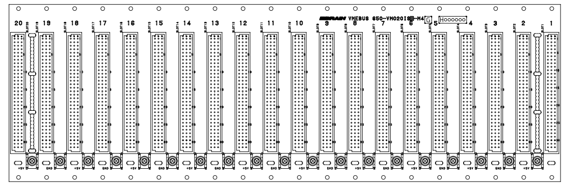
半田面視
